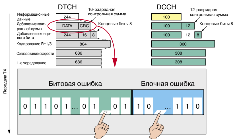
Вставка в выходной сигнал битовых и блочных ошибок
